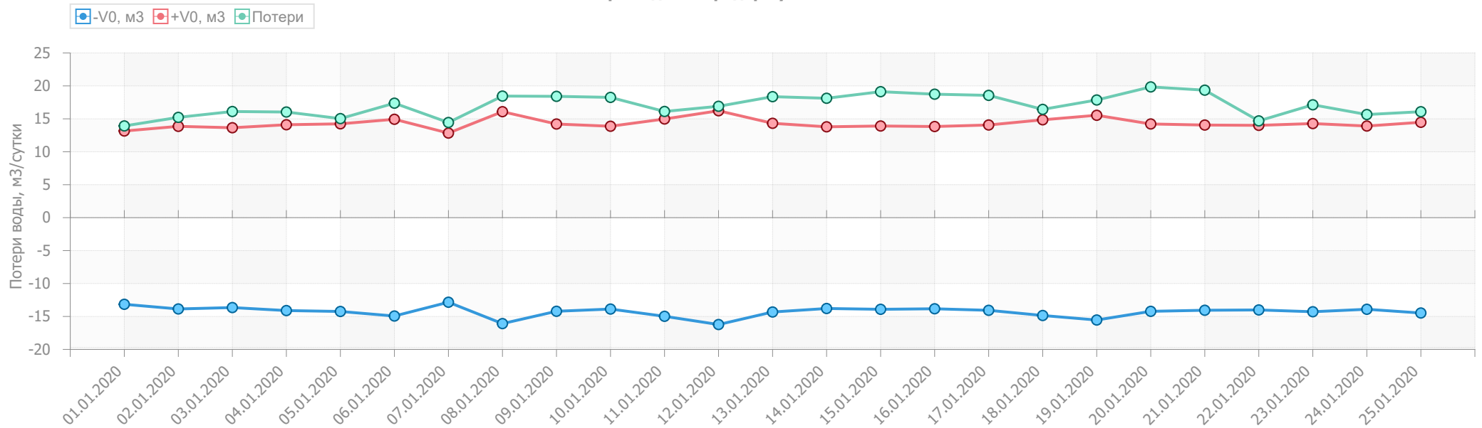
Потери воды и коридор нулевого баланса
