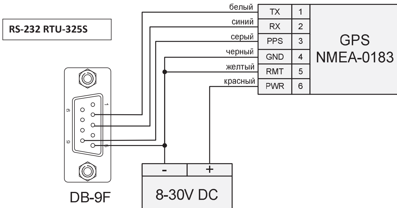
Рисунок Г.2 - С использованием импульсного выхода PPS
