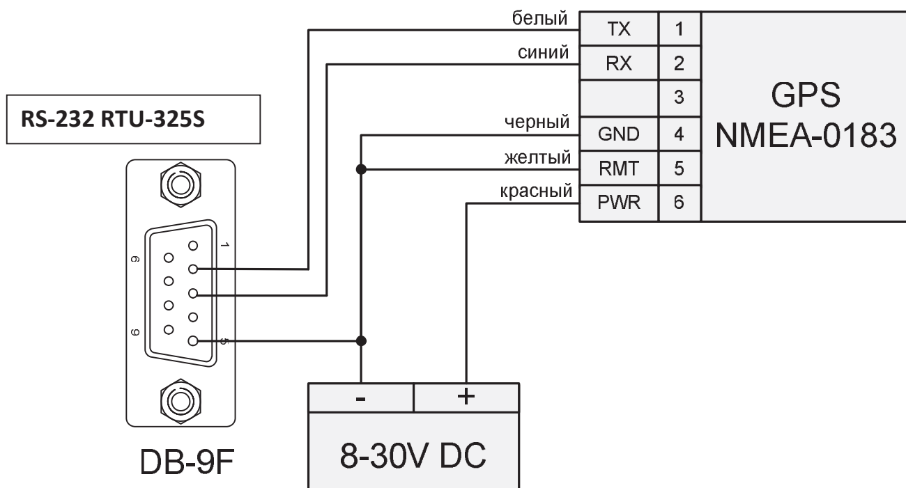
Рисунок Г.1 - Без использования импульсного выхода PPS
