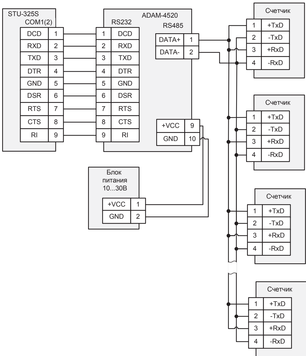
Рисунок Д.2 - 2-х проводная схема
