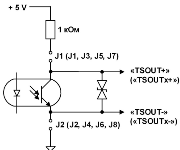
Рис.Ж.1. Схема оконечного каскада универсальных выходов.
