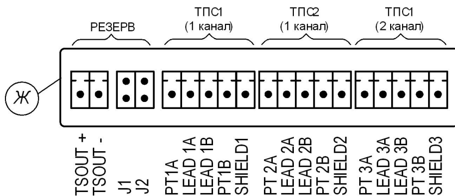
Рис.Е.4. Коммутационные элементы модуля температурных входов.
