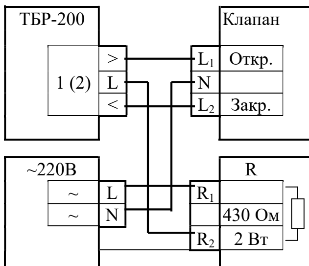
Рисунок 3.6 – Схема подключения исполнительных механизмов с пусковым током, превышающим порог защиты от КЗ ( 0,5\text{А} ), к регуляторам серии 0001.
