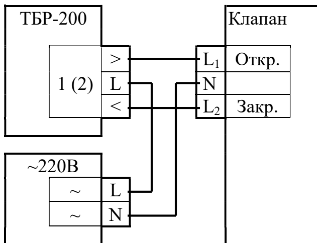
Рисунок 3.5 – Схема подключения исполнительных механизмов
