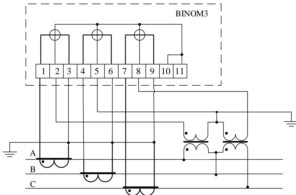
Рисунок 18.10 – Схема включения счетчика «BINOM3» в трехфазную трехпроводную сеть
