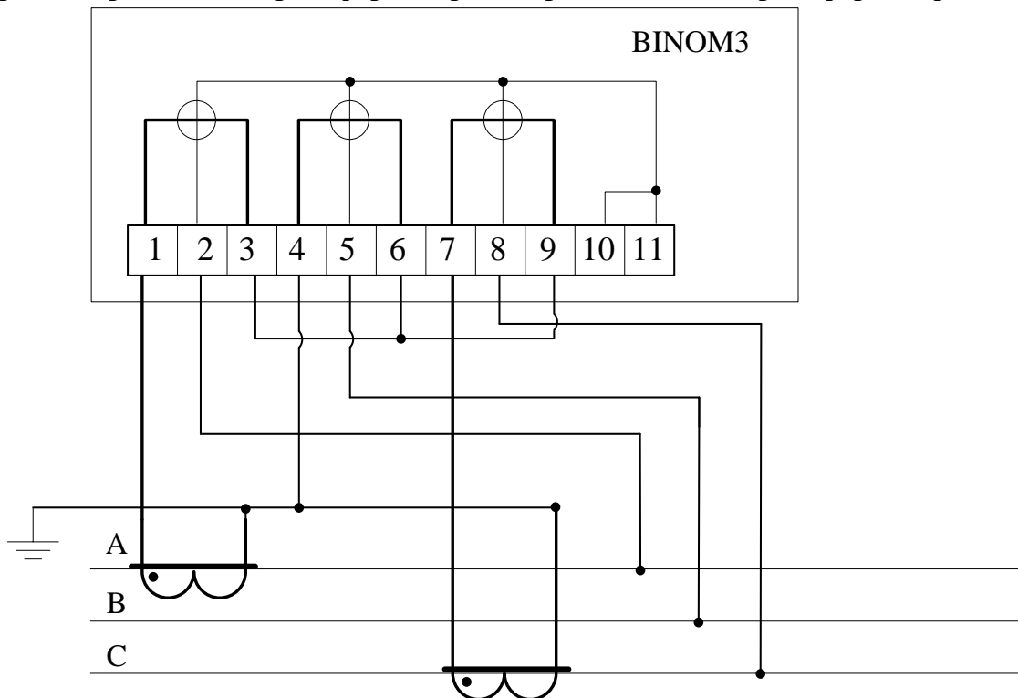
Рисунок 18.6 – Схема включения счетчика «BINOM3» в трехфазную трехпроводную сеть через измерительные трансформаторы напряжения и два трансформатора тока.
