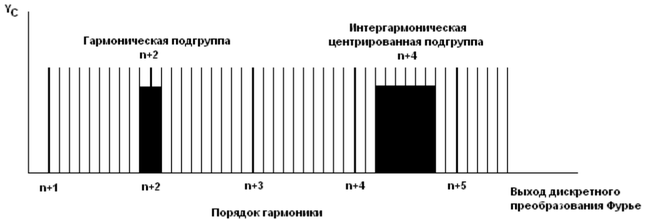
Рисунок 5 – Схема образования гармонических подгрупп и интергармонических центрированных подгрупп
