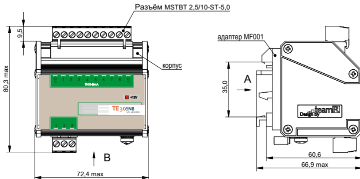
Рисунок 16 – Габаритный чертеж блока «TE305N8»
