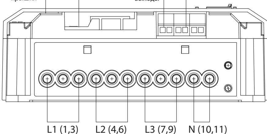
Схема подключения фазных проводов
