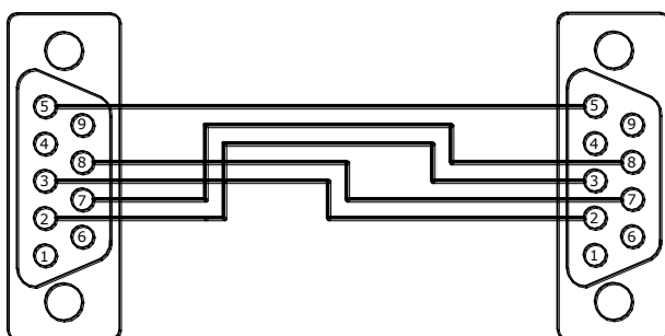
Рис. 6.3 Нуль - модемный кабель RS-232
