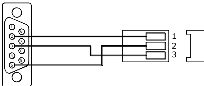
Рис. 6.2 Переходной кабель RS-232 (104/106 - АД)
