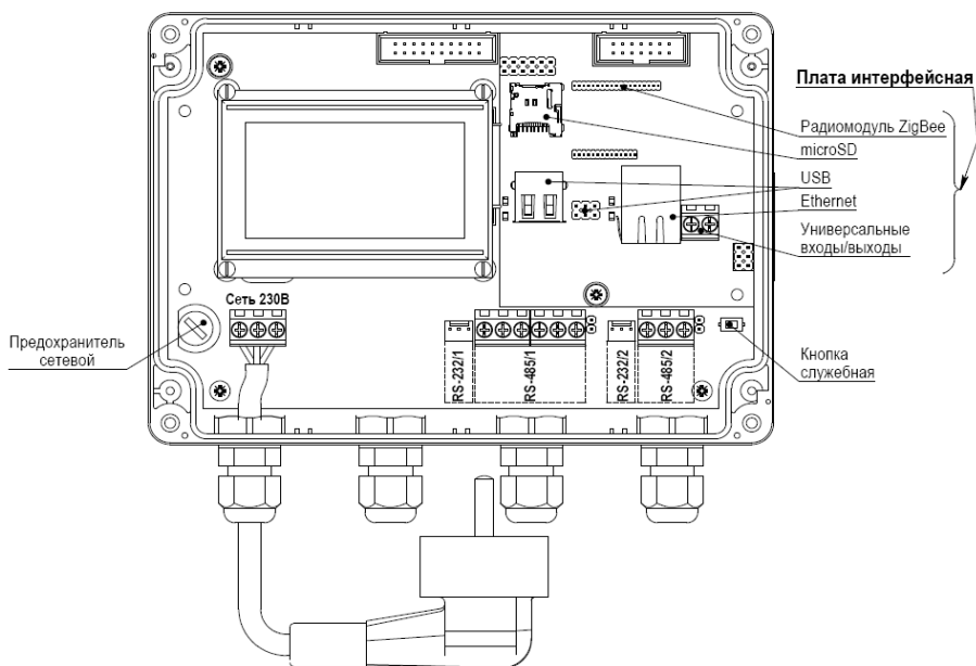
Рис. 6.1 Вид ТСМ-И со снятой крышкой
